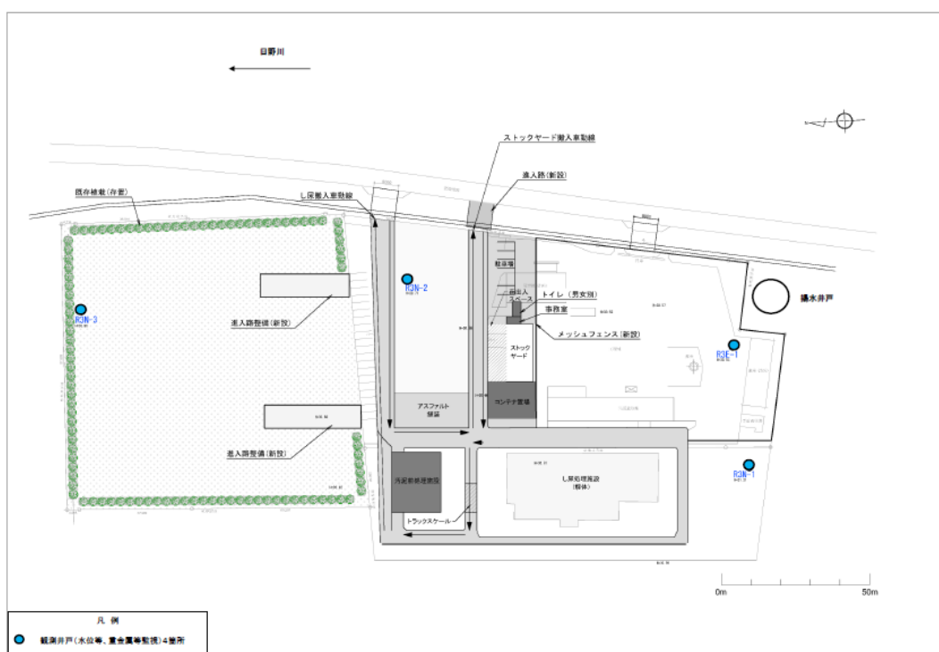
図 地下水モニタリングの調査地点位置図
